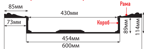
KS61A-18D рама: 600x600x25, короб: 454x454x89
