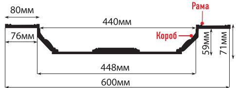
КС61-56 рама: 600x600x12, короб: 448x448x59
