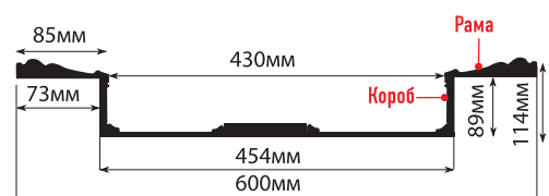
KS61A-19D рама: 600x600x25, короб: 454x454x89
