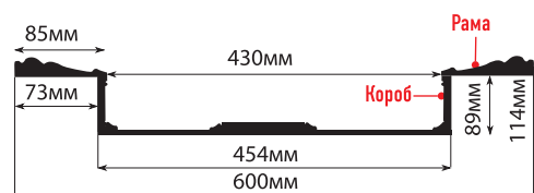
K561A-57 рама: 600x600x25, короб: 454x454x89
